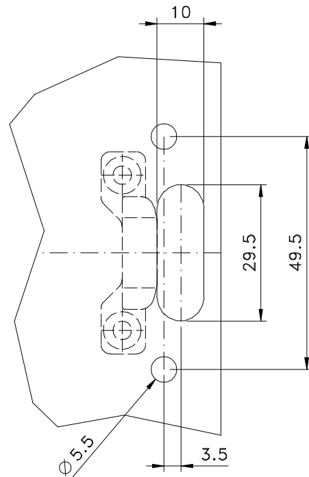
DETALHE - USINAGEM FECHO
