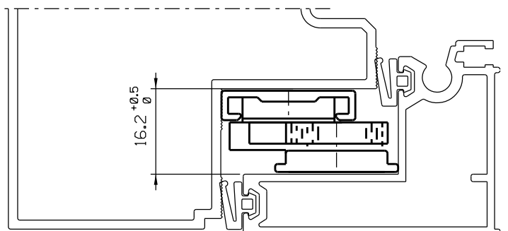
Instalação - escala 1:1
