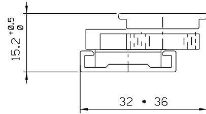
Vista - escala 1:1
