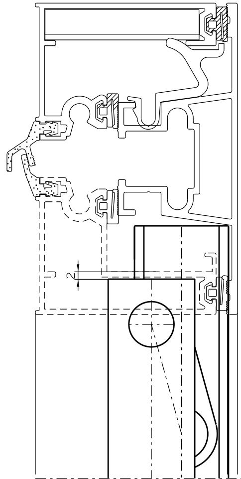
Vista - escala 1:1
