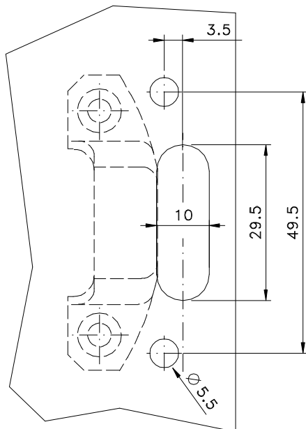
Detalhe para instalação. ESCALA 1:1
