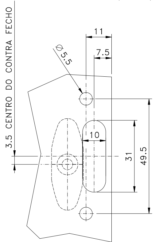
USINAGEM ESCALA 1:1
