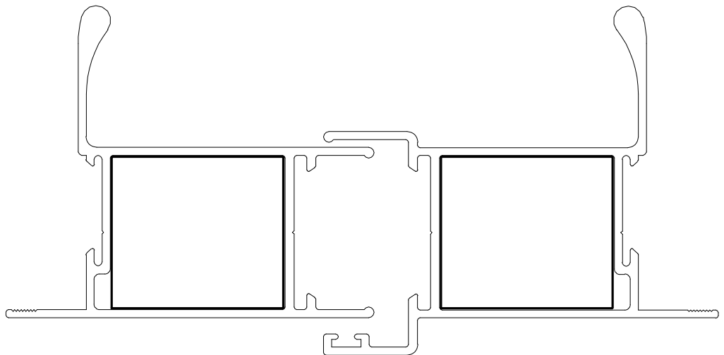
Instalação - escala 1:1
