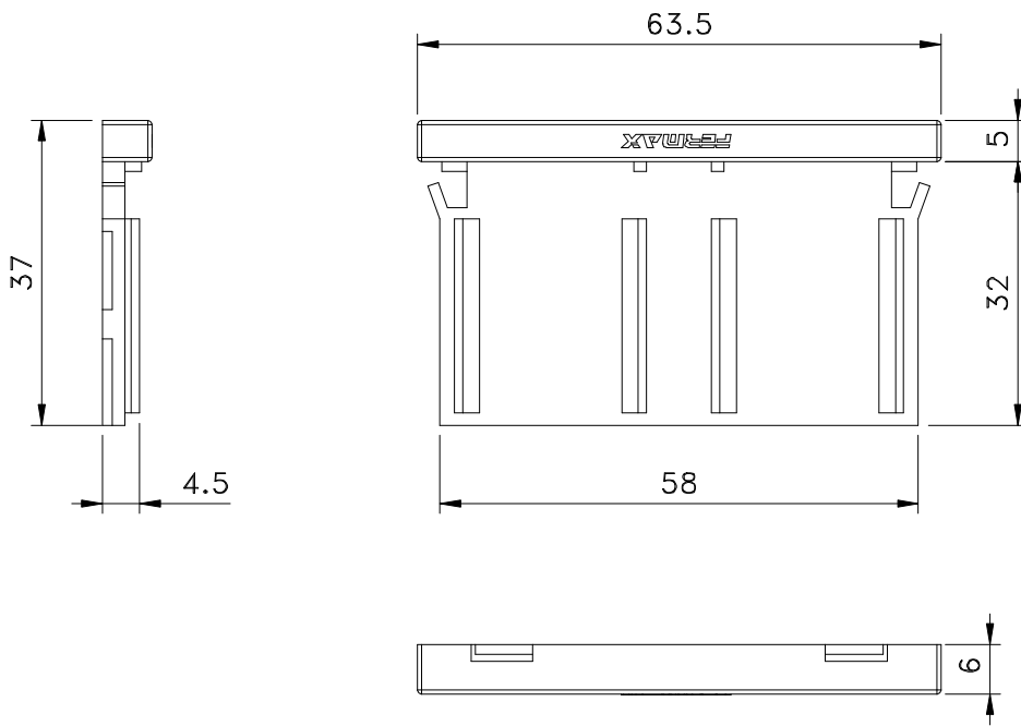
Vistas - escala 1:1
