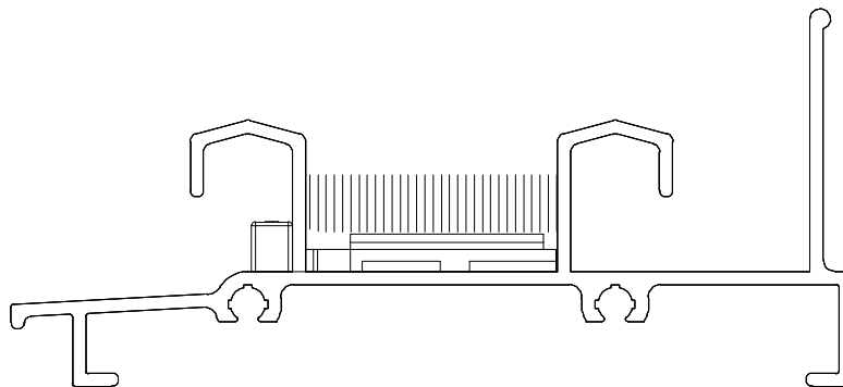
Instalação - escala 1:1
