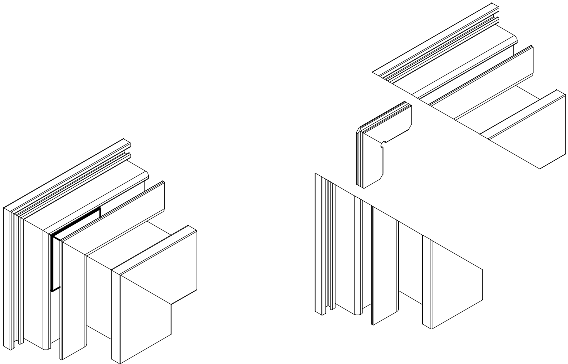
DETALHE DE APLICAÇÃO - sem escala
