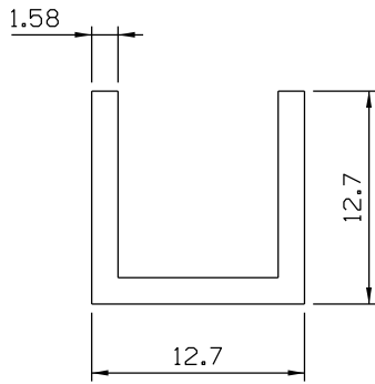
TRILHO GUIA 1/2" 0,153 Kg/m linear
