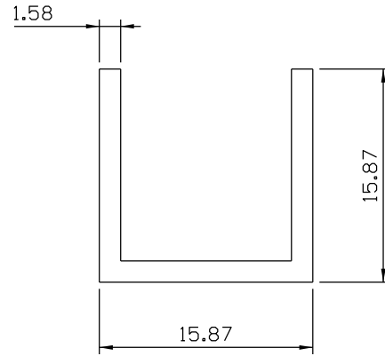
TRILHO GUIA 5/8" 0,175 Kg/m linear
