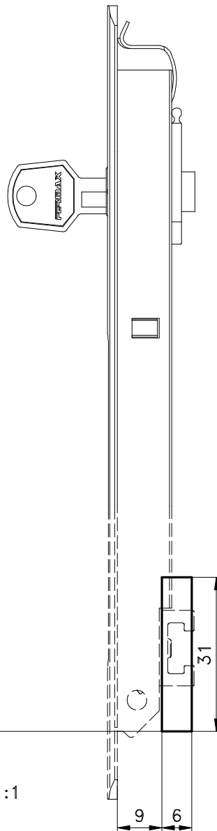
Vistas - escala 1:1
