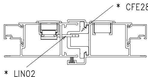
Instalação - escala 1:2
